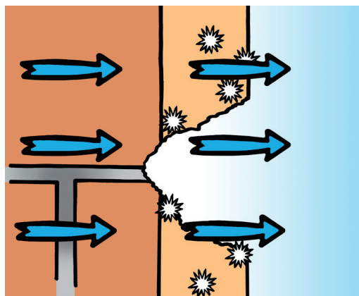
destrukční krystalizační proces
